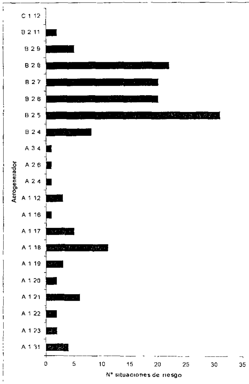
Figura 7. Situaciones de riesgo para las aves detectadas en los distintos aerogeneradores del parque eólico de Guerinda.
