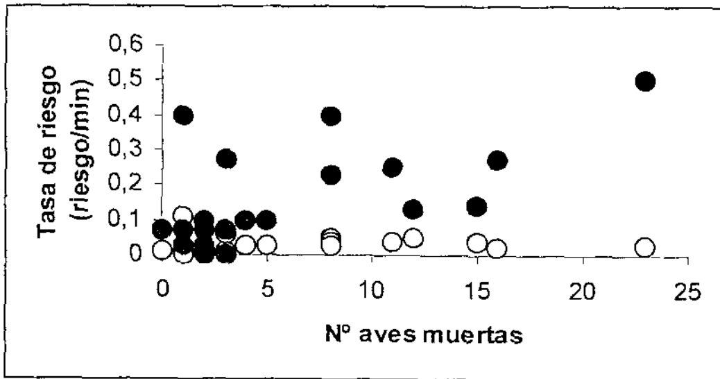
Figura 10. Relación existente entre el número de aves muertas por colisión y la tasa media de riesgo (círculo blanco) y la tasa de riesgo máxima (círculo negro) detectada en los distintos puntos de control situados en los parques eólicos estudiados.
