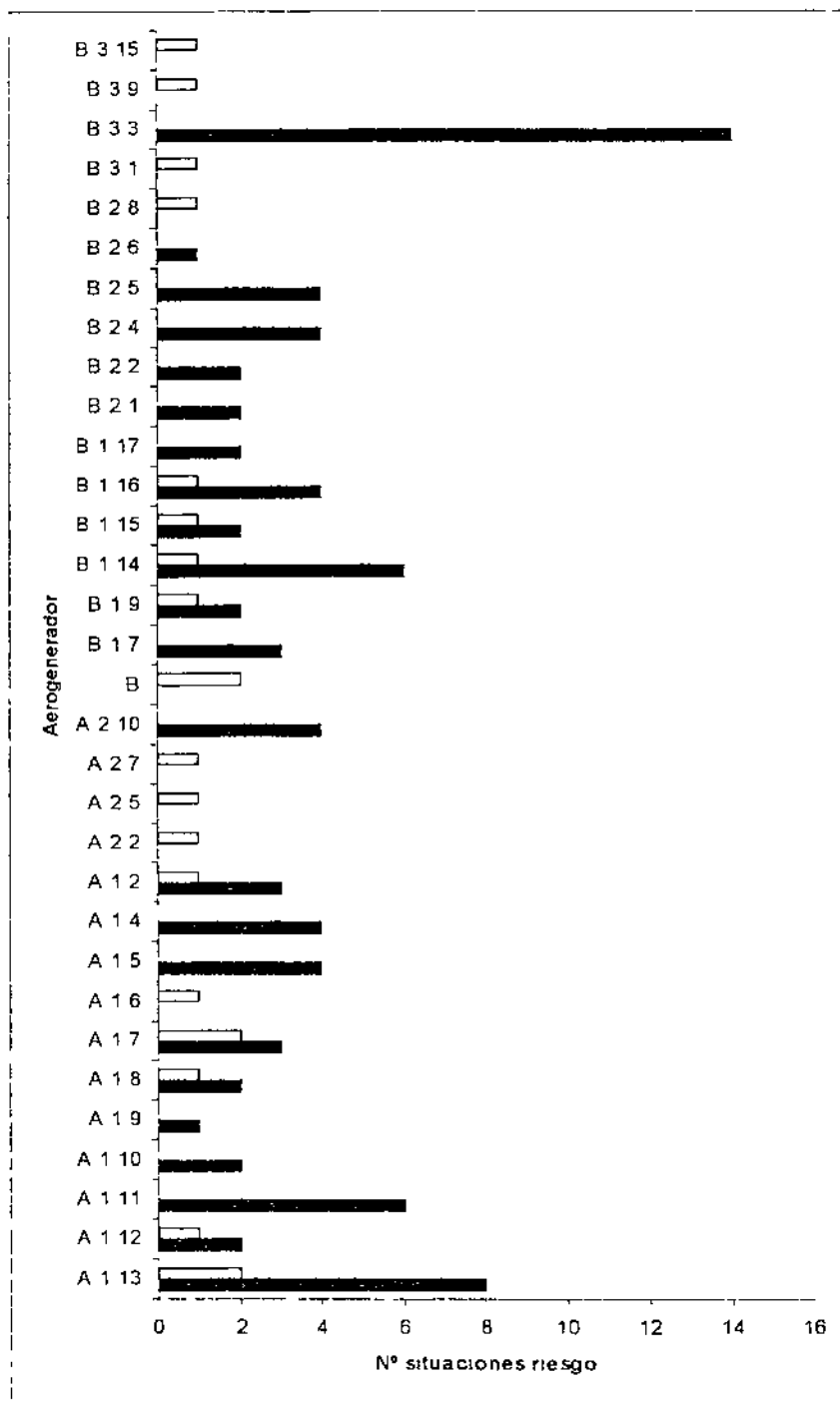
Figura 12. Relación entre el número de situaciones de riesgo (barras negras) detectadas en el parque eólico de Izco-Aibar y el número de aves localizadas muertas (barras blancas).
