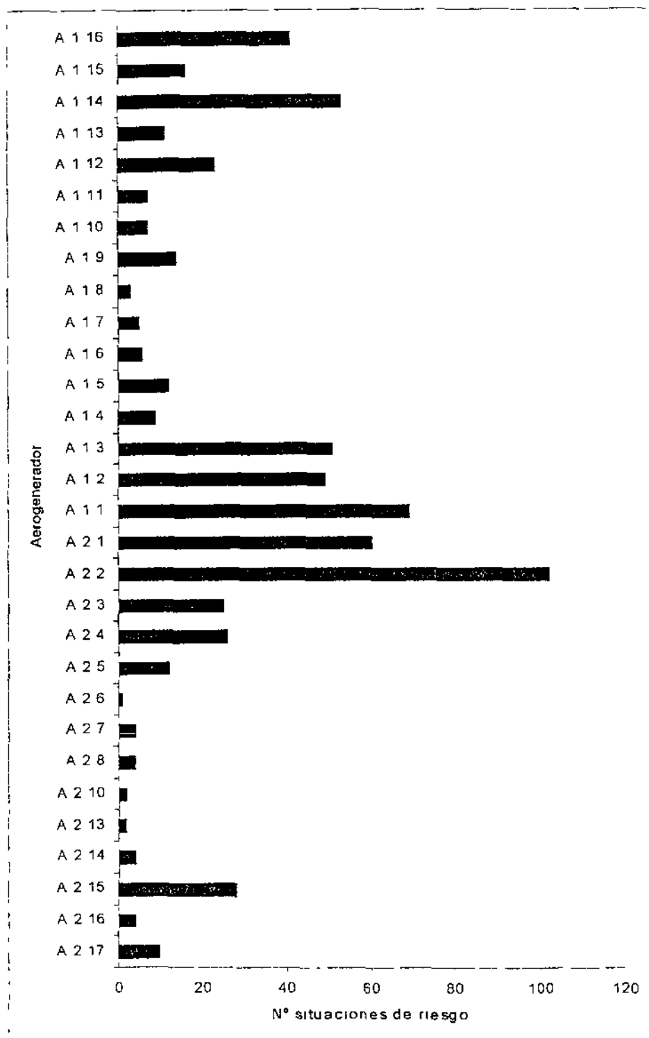
Figura 4. Número de situaciones de riesgo detectadas en cada uno de los aerogeneradores del parque eólico de Salajones.
