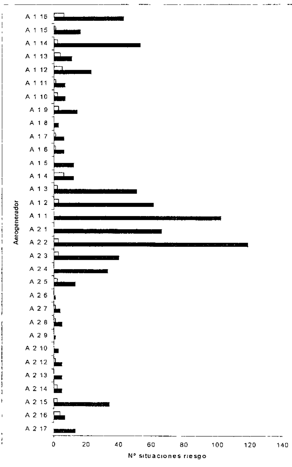
Figura 11 Relación entre las situaciones de riesgo (barras negras) detectadas en el parque eólico de Salajones y el número de aves localizadas muertas (barras blancas)
