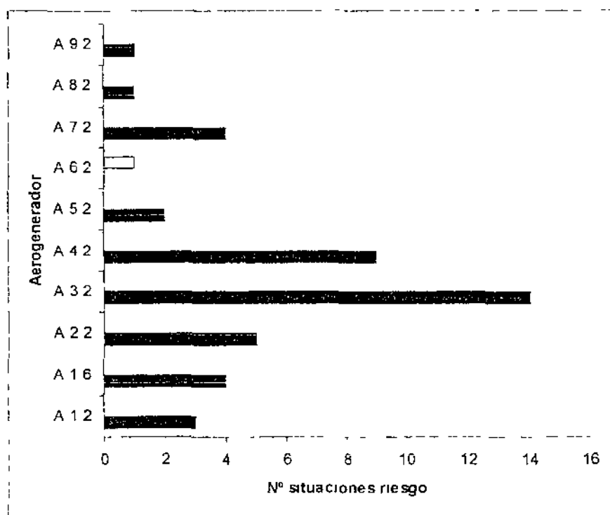
Figura 16. Relación entre las situaciones de riesgo (barras negras) detectadas en el parque eólico de Leitza-Beruete y el número de aves muertas localizadas (barras blancas)
